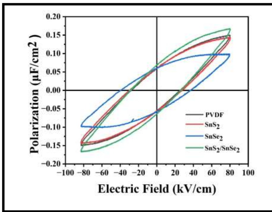
Fig. 8: PE hysteresis loop.
