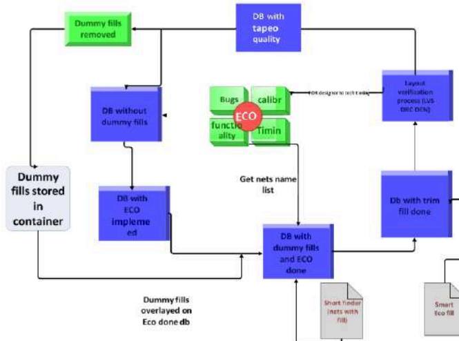
Fig. 4.1 Smart ECO fill process
